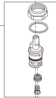
RP78871 Stem Unit Assembly, Seat & Spring, Bonnet Nut & Washer Ensamble de la Unidad del Vástago, Asiento y Resorte, Bonete y Arandela Obtuteur, siège et ressort, écrou à chapeau et rondelle
