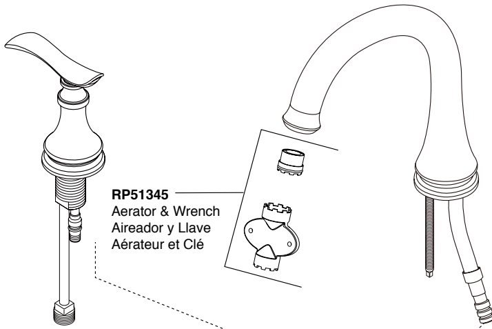
RP78871 Stem Unit Assembly, Seat & Spring, Bonnet Nut & Washer Ensamble de la Unidad del Vástago, Asiento y Resorte, Bonete y Arandela Obtuteur, siège et ressort, écrou à chapeau et rondelle
